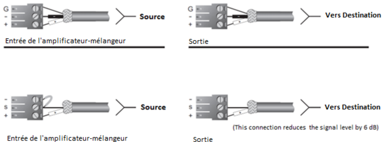
[Figure 2.5 Câbles d'entrée et connecteurs]
