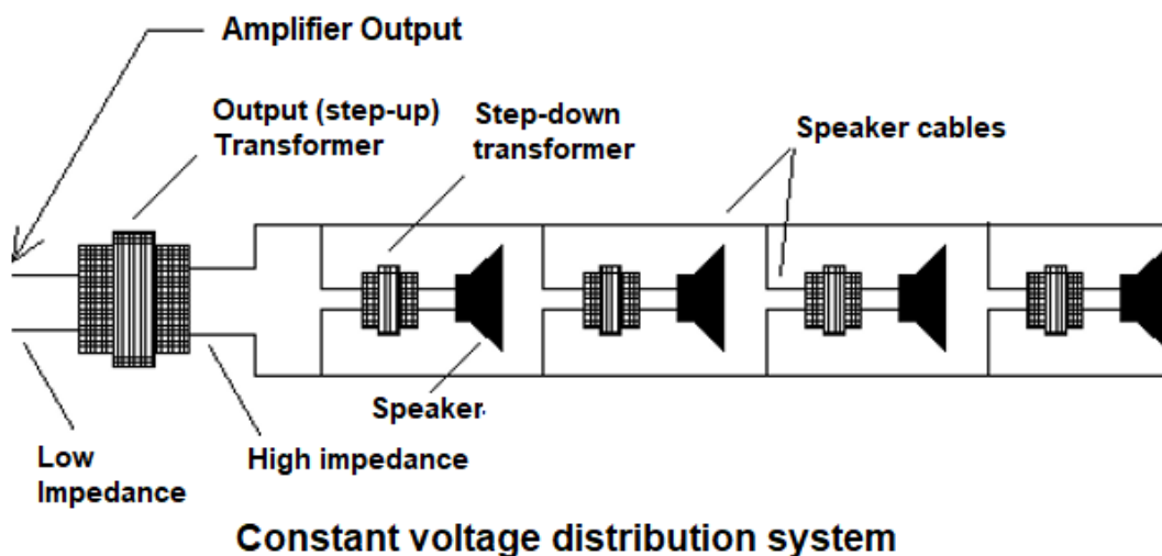
[Figure 2.3 Branchement de haut-parleur à tension constante]
