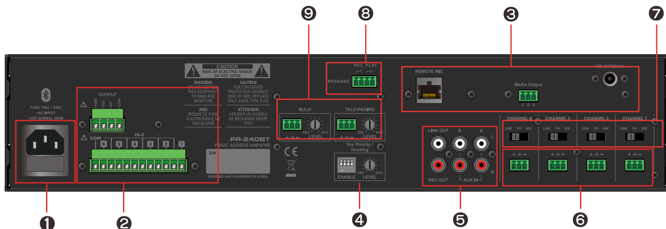
[Figure 1.2 Schéma du panneau arrière]
