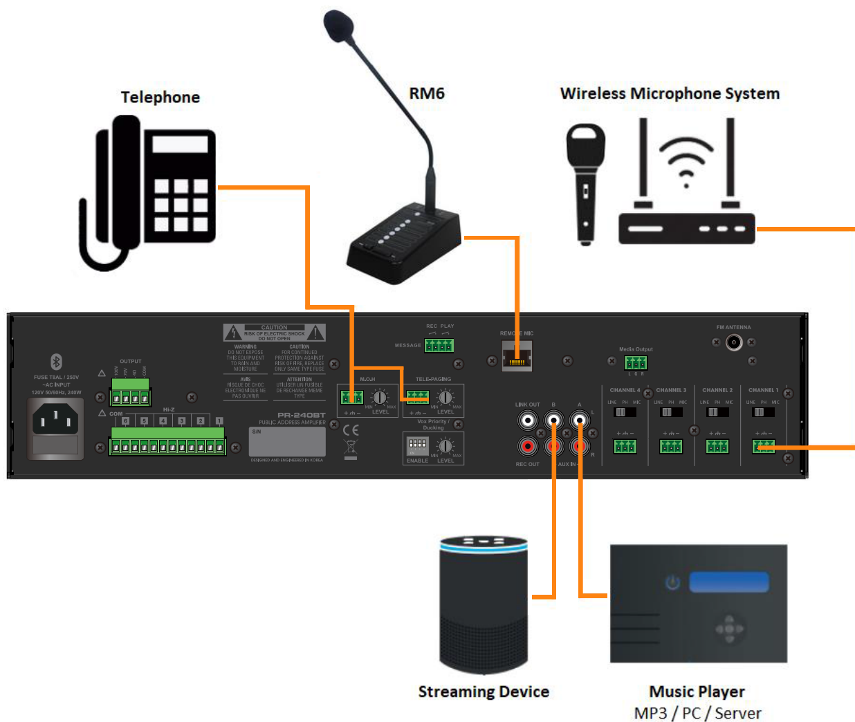
[Figure 2.4 Exemple de branchement]
