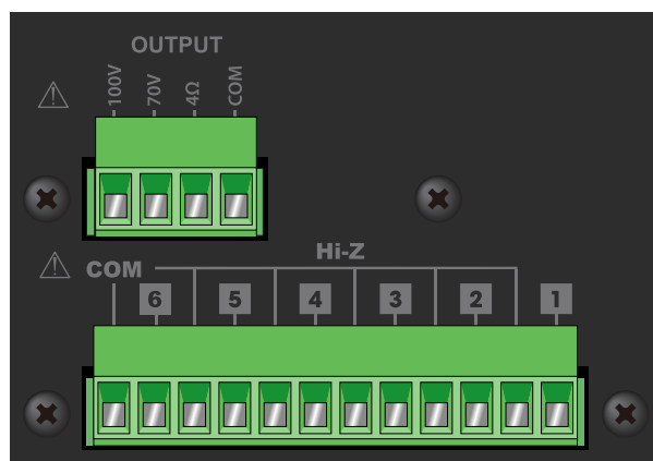
[Figure 2.3 Connecteurs de sortie de haut-parleur]
